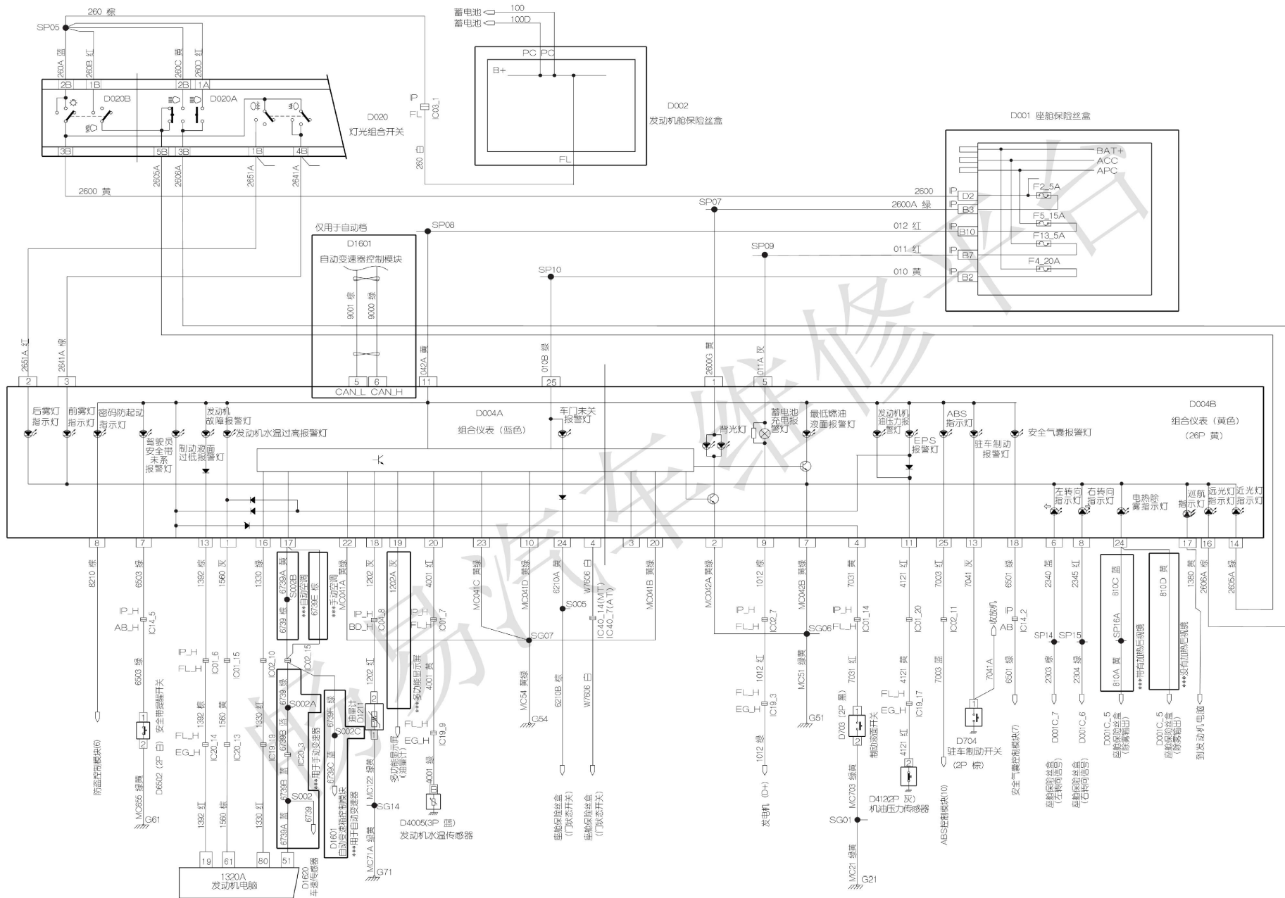
组合仪表电器原理图
